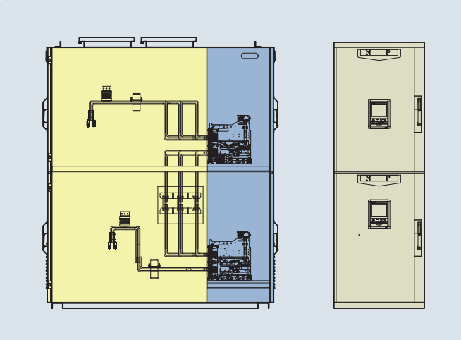
480V 저압반
